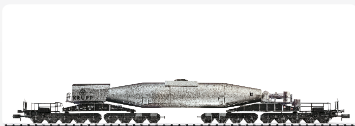
15553 Torpedopfannenwagen 119,99* € III-IV Torpedo Ladle Car
